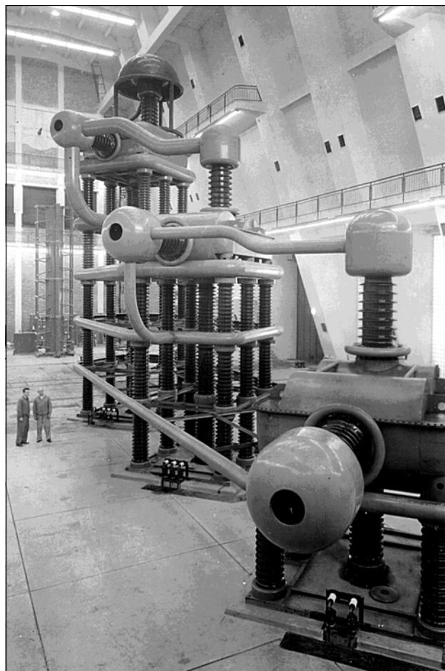
Kaskádní transformátor TuR těsně před spuštěním zkušebního provozu (jaro 1954).
