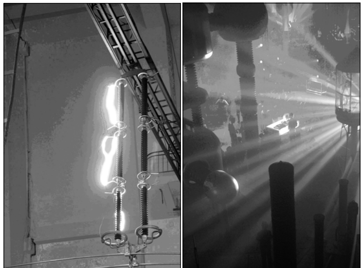
Střídavý přeskok na dvojitém nosném izolátoru.
