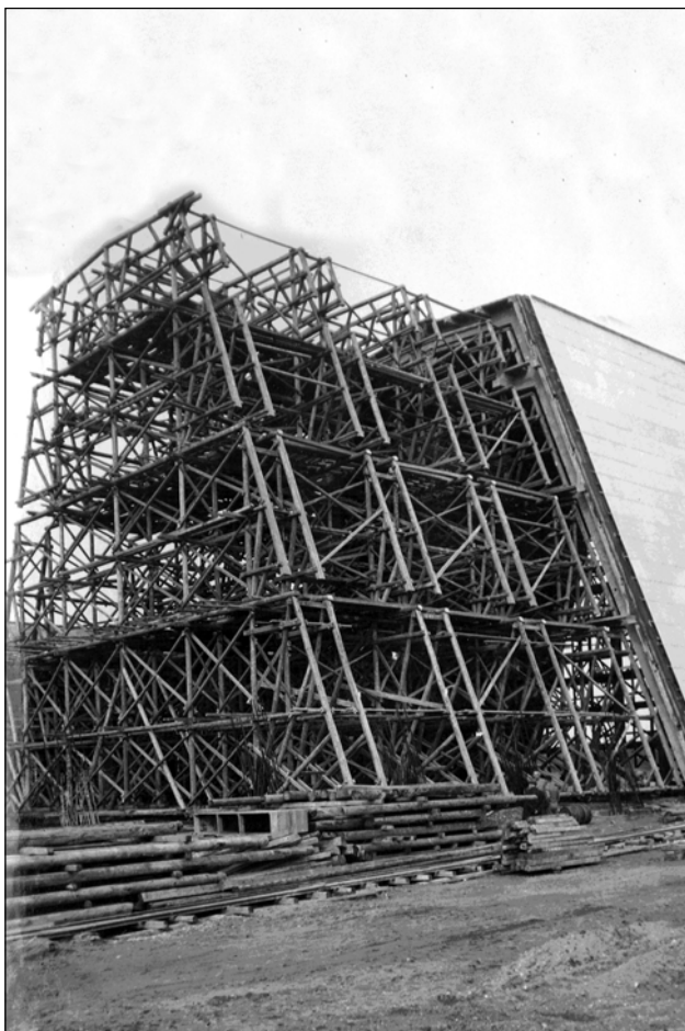
Stavba probíhala ojedinělou technologií, kdy dřevěné lešení ukotvené na kolejích bylo postupně přesouváno.
